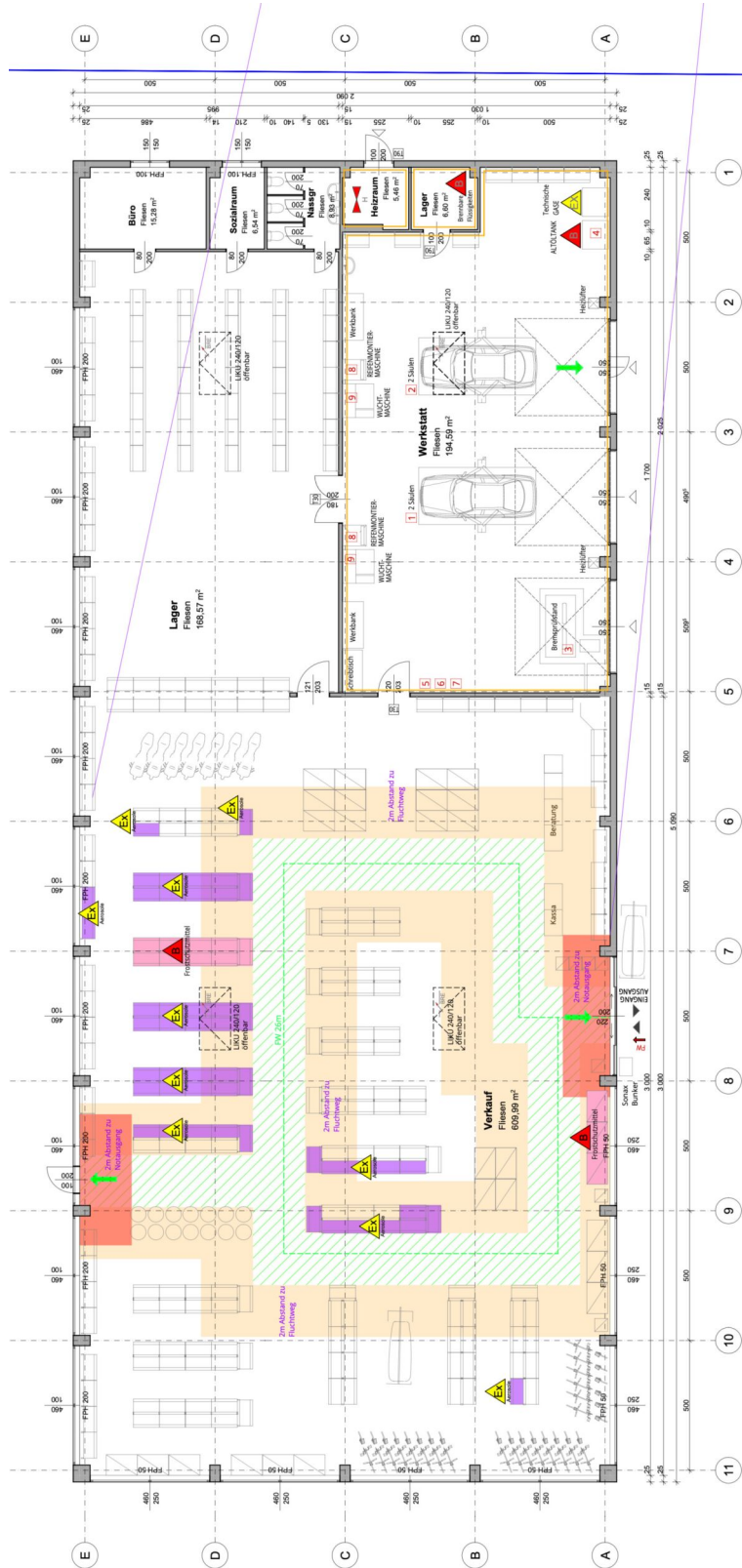
GRUNDRISS ERDGESCHOSS M 1:100
